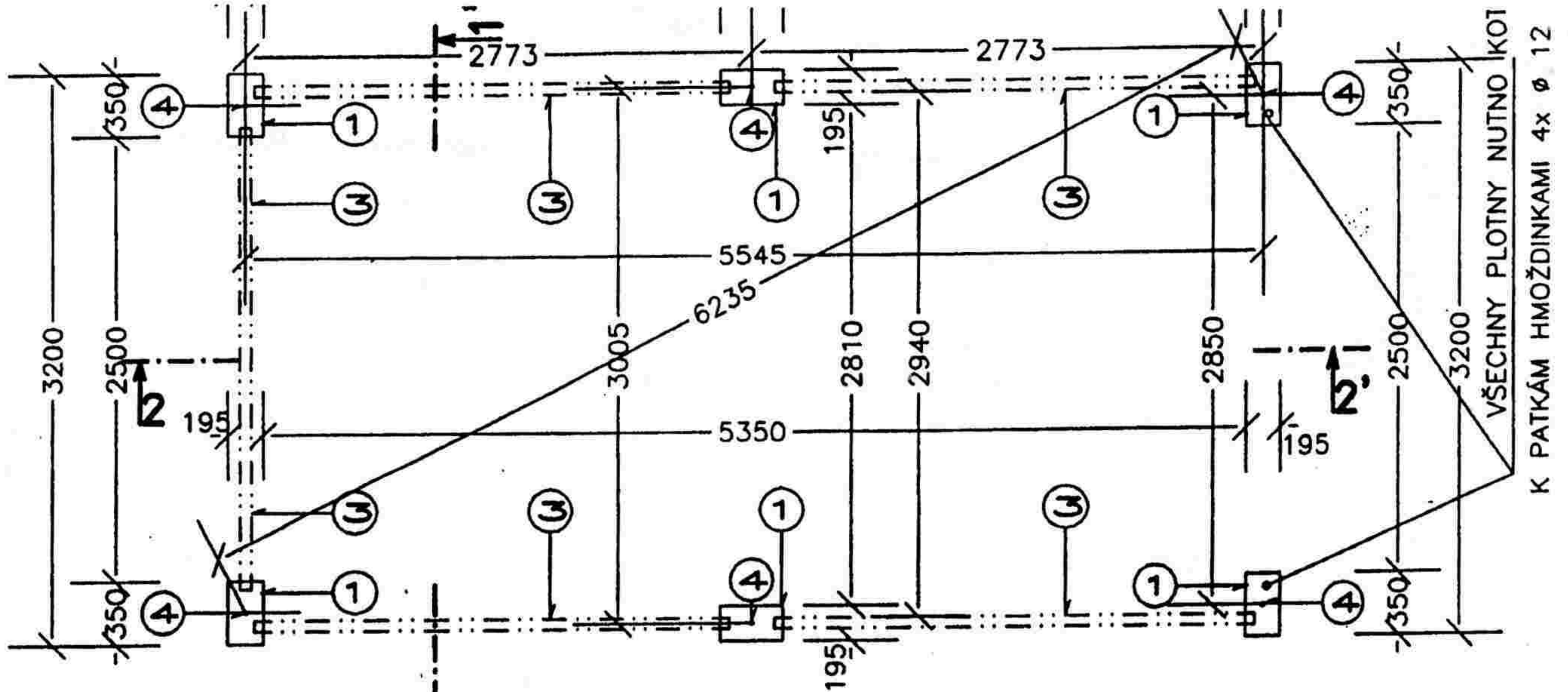
PŮDORYSNÉ SCHEMA OSAZENÍ KOTEVNÍCH PLOTEN
