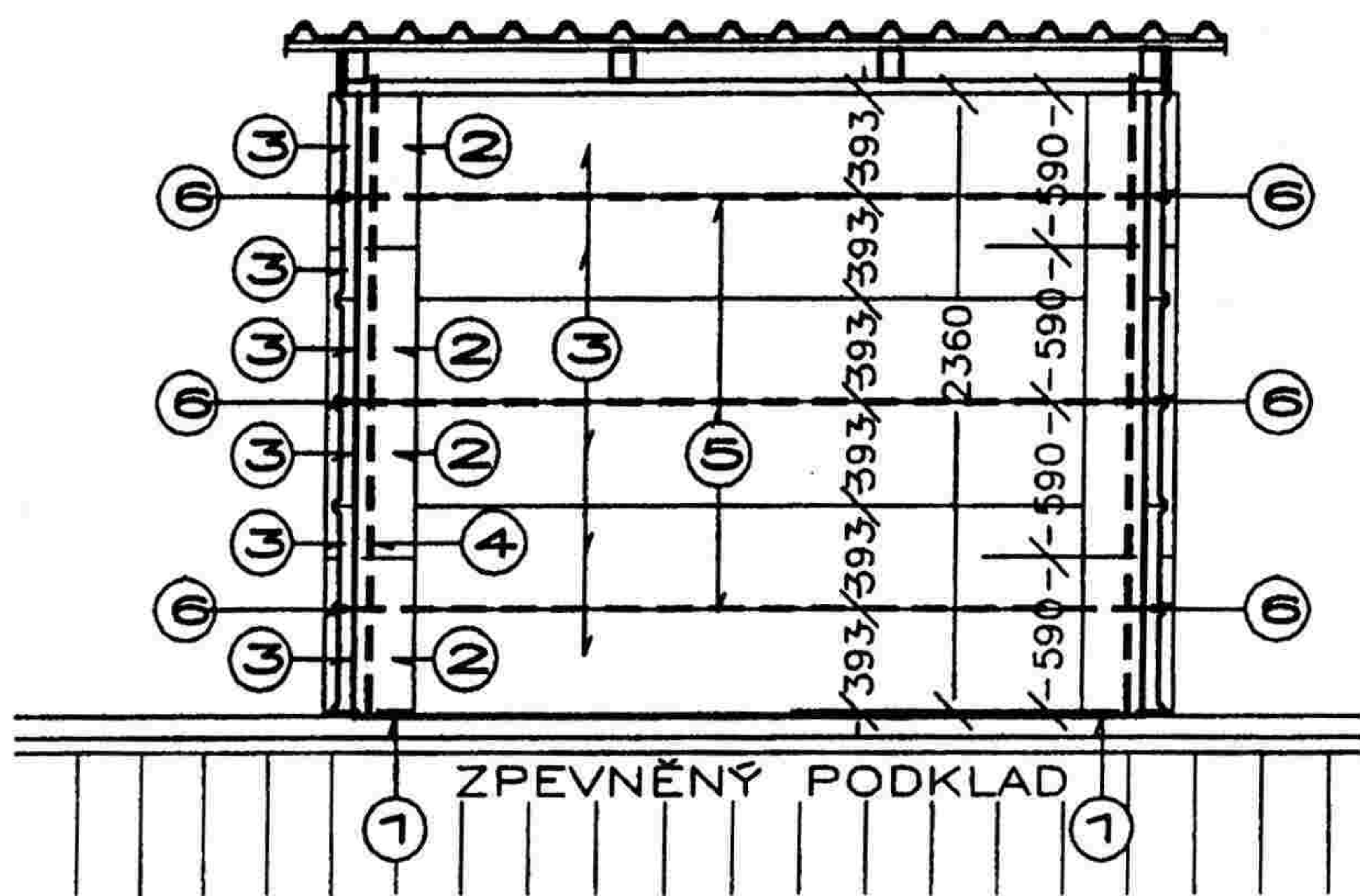
PŘÍČNÝ ŘEZ : 1-1'
