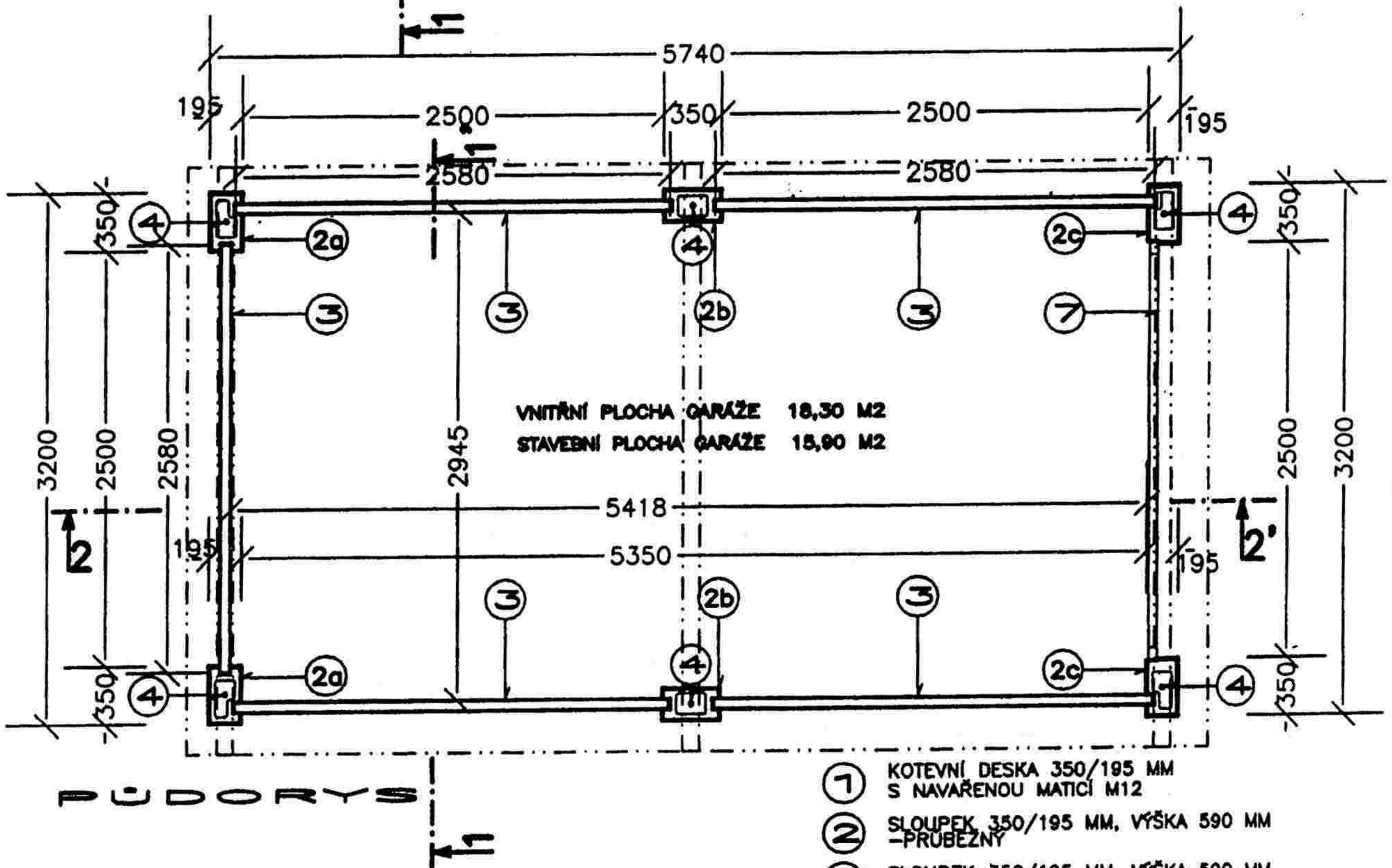
PŮDORYSNÉ SCHEMA OSAZENÍ KOTEVNÍCH PLOTEN
