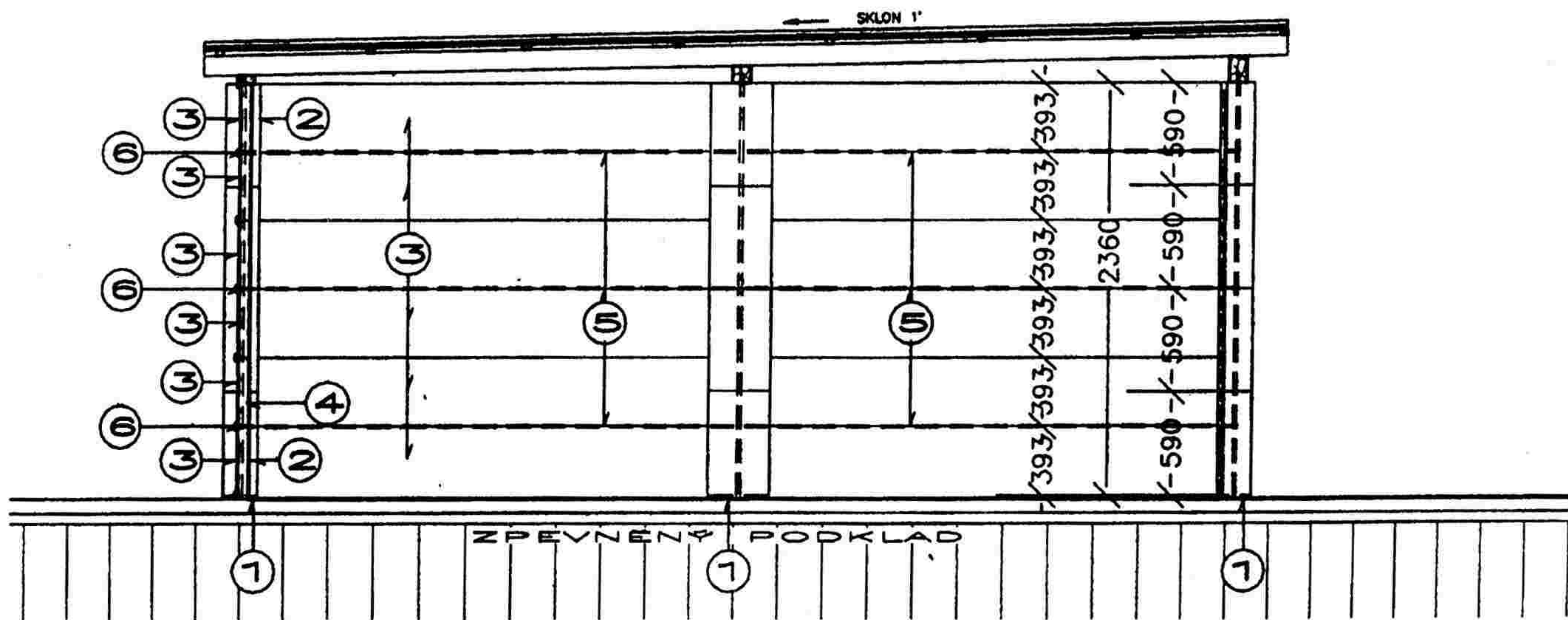
PODELNÝ ŘEZ : 2-2'
