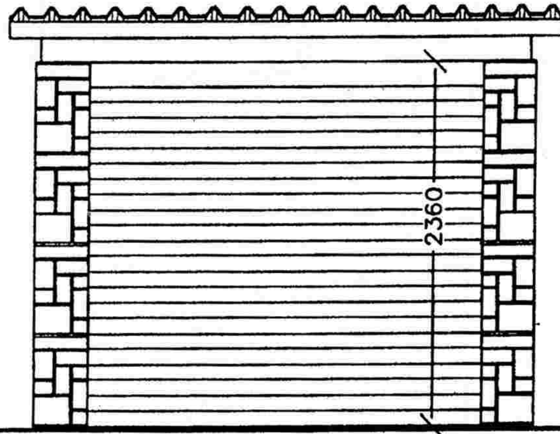
ČELNÍ POHLED
